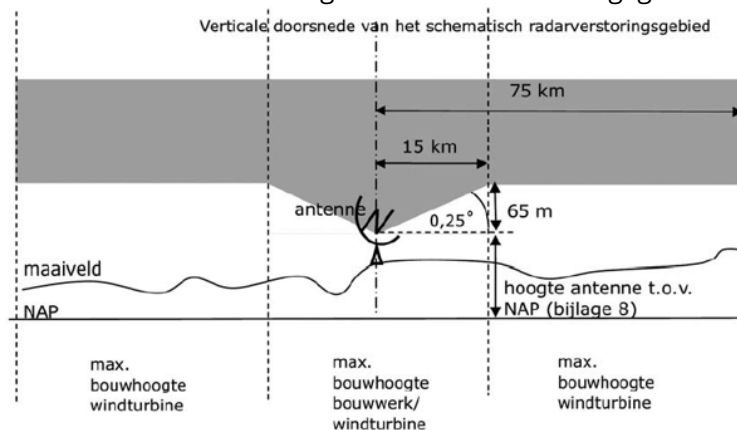
Schematische weergave bouwhoogte i.r.t. radarverstoring
